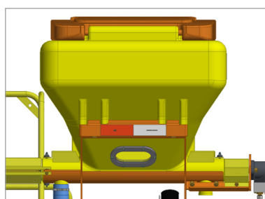
Caja de Abono con capacidad de 270 litros cada una, con visor transparente para verificación del nivel de abono.
