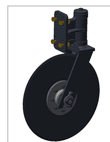
Disco de corte de 26" y con 3 reglajes de altura para mayor ajuste de corte.
