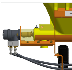
Sistema de transmisión directa del motor, eliminando cadenas y engranajes reductores.
